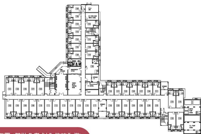
1/F樓平面圖 (僅供參考;以入住時為準)
